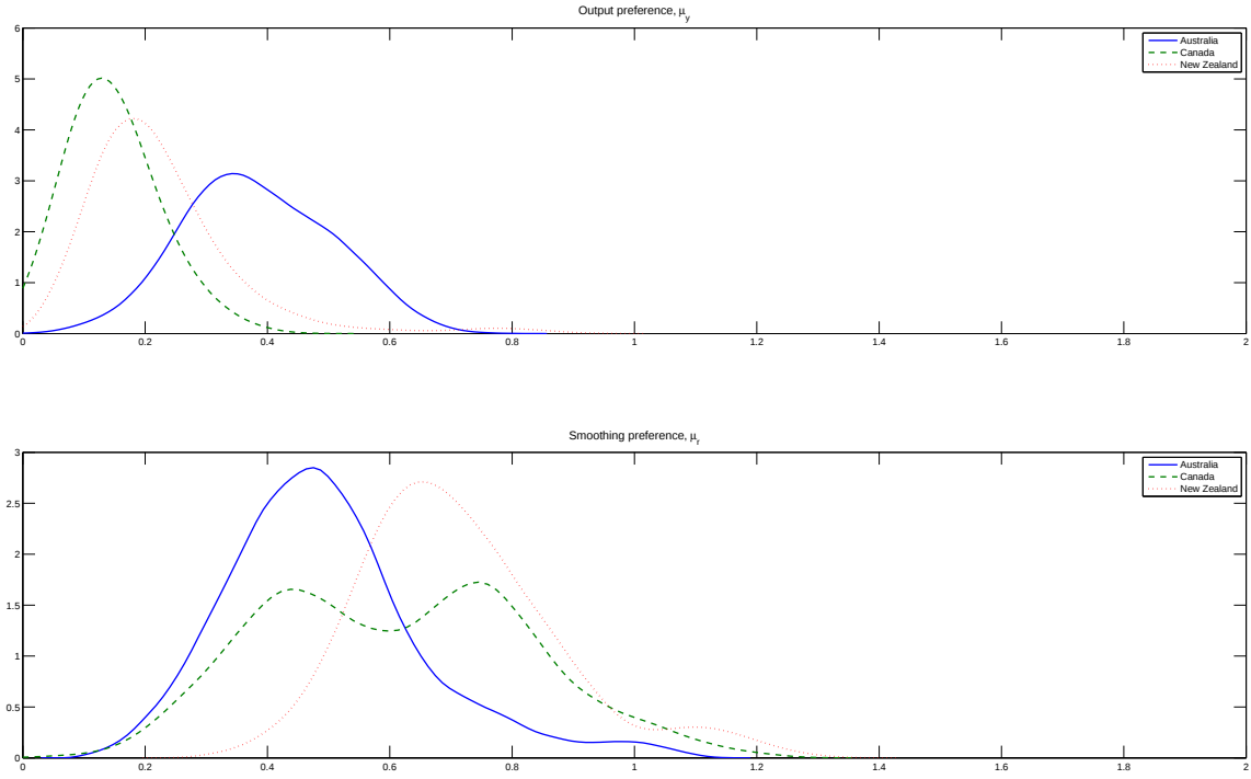
Fig. 4. Posterior comparison of loss function parameters
